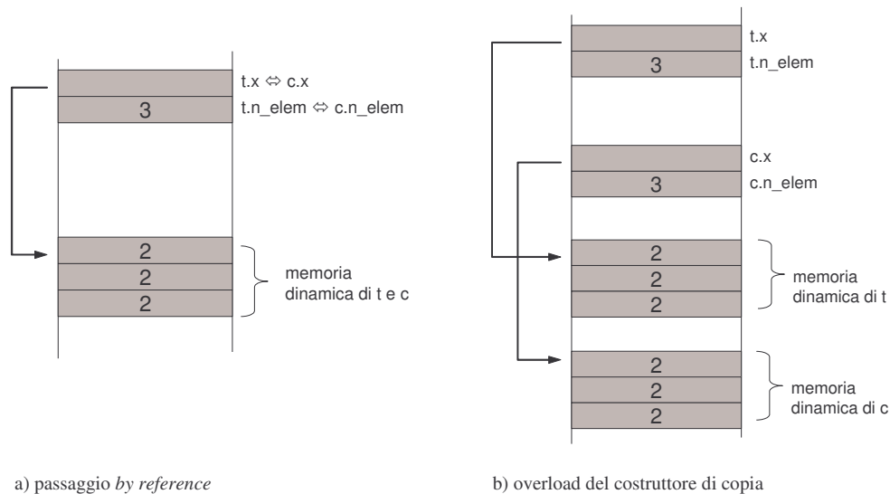
Figura 8. a) Passaggio by reference: t e c coincidono (anche se c è dichiarato di tipo const e pertanto non può essere modificato). b) Overload del costruttore di copia: c e t sono due oggetti identici ma distinti .
